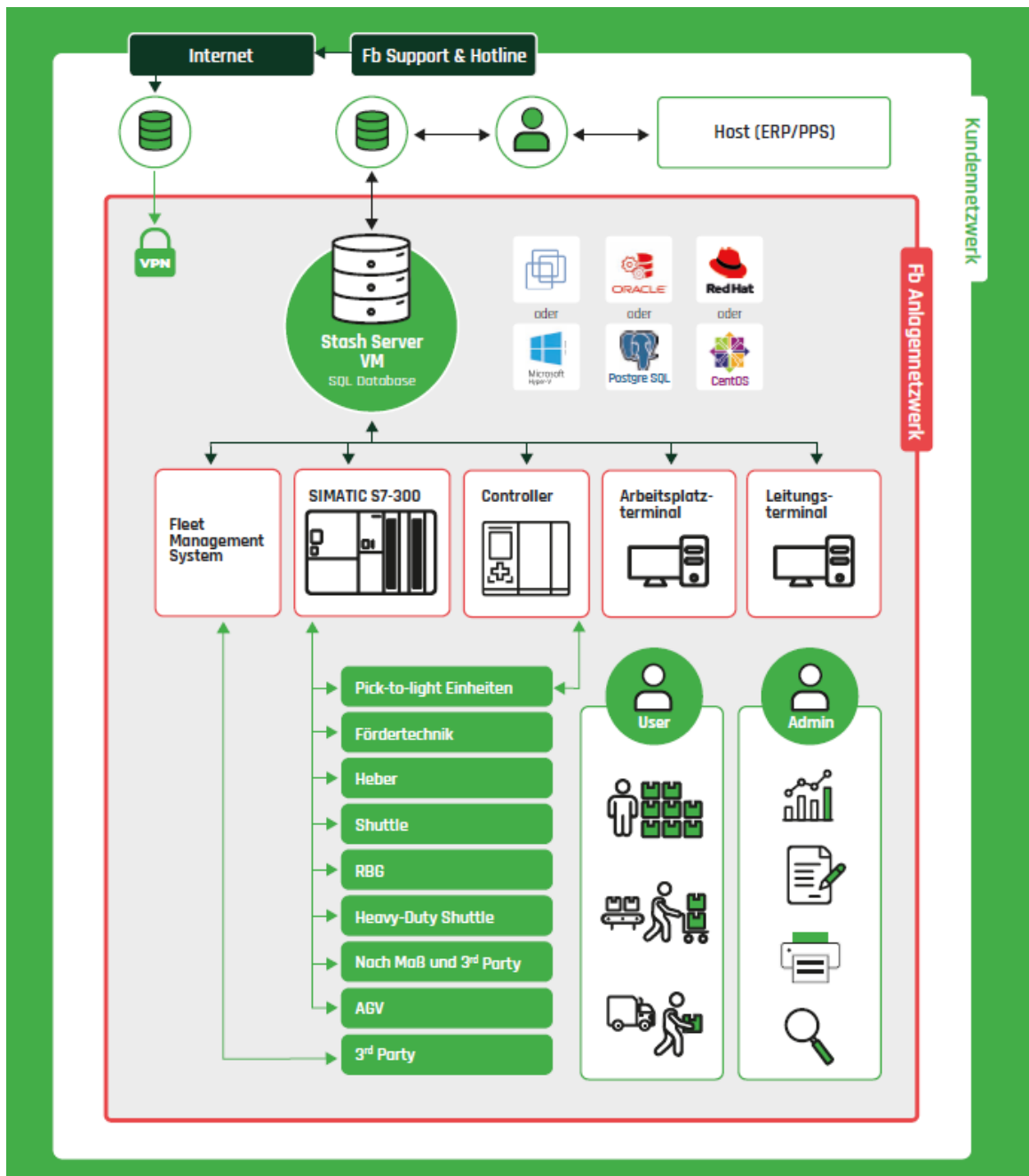
Abbildung 1: Stash im Einsatz in einer Anlage
